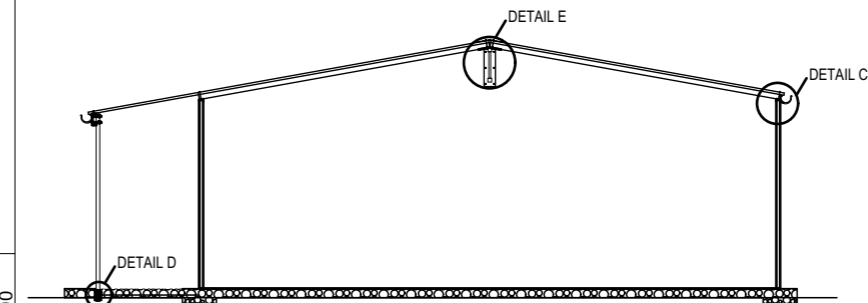
SECTION E - E
